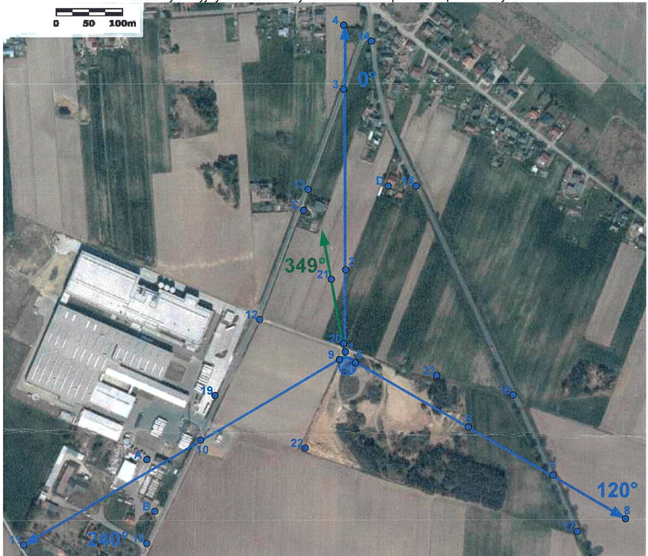
Szkiec sytuacyjny z zaznaczonymi kierunkami i punktami pomiarowymi
